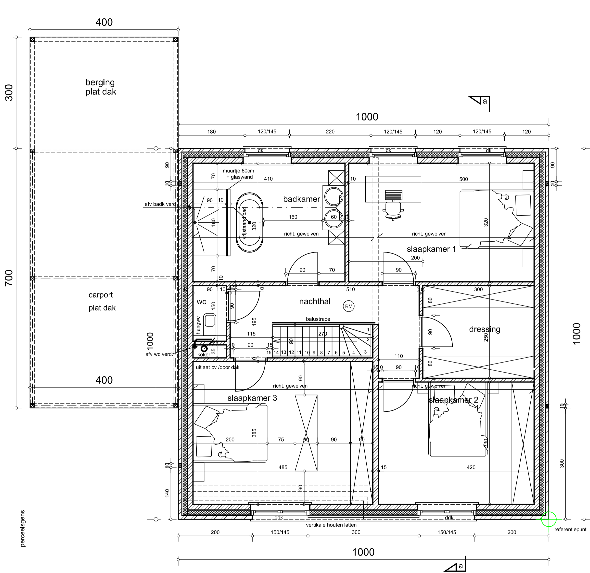
verdieping / 1:50
